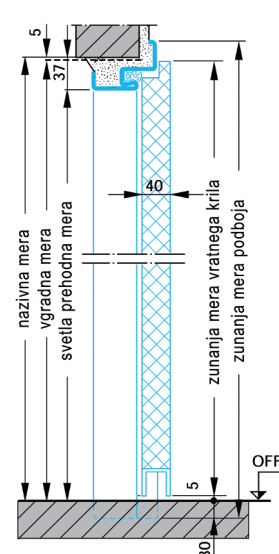
VERTIKALNI PREREZ
