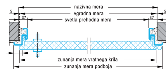
HORIZONTALNI PREREZ
