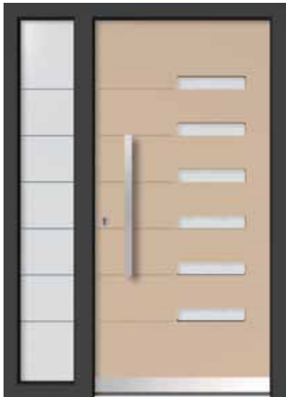
ST 100 T 213 steklo z motivom .....PESKANO MS 66A držalo 75 cm .....D 200 odkapni profil .....E 75 kriilo .....RAL 1015 podboj .....RAL 7016
