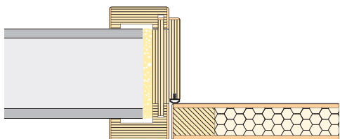
Podboj in krilo v isti ravnini Skrita nasadila
