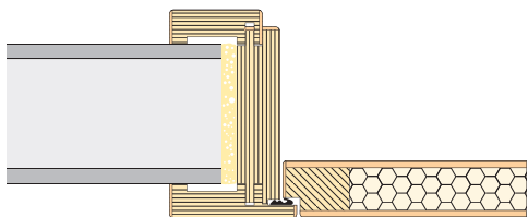
Podboj in krilo v isti ravnini Skrita nasadila, odpiranje čez podboj
